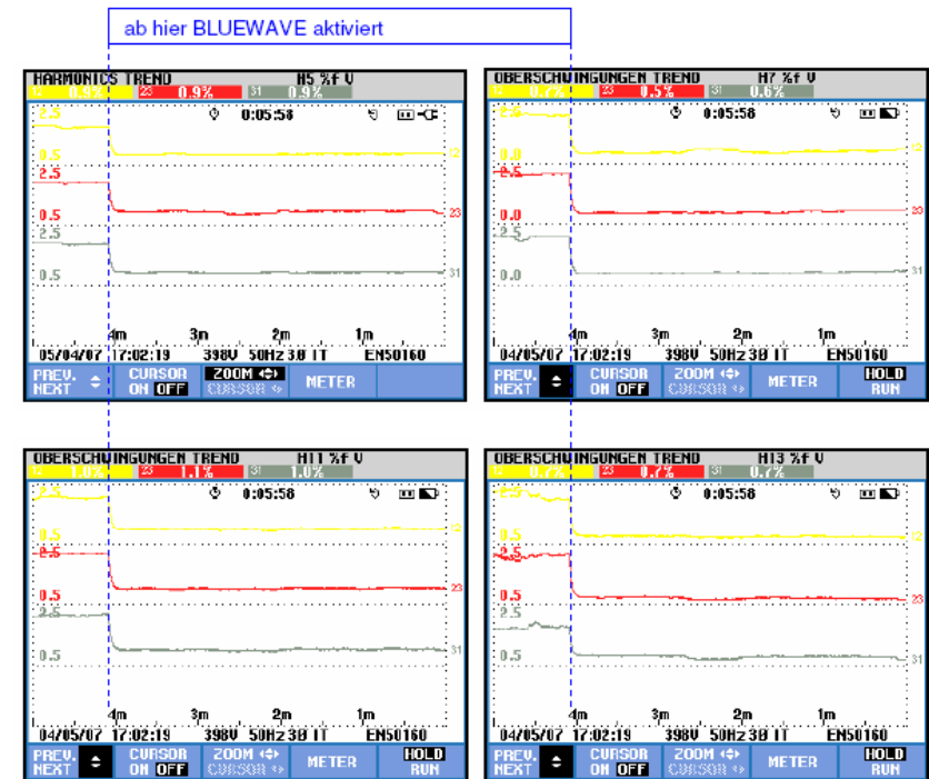
Abb. 4: Trend der Spannungsüberschwingungen 5., 7., 11. und 13. Harmonische (BLUEWAVE ist ab blauer Linie aktiviert)
