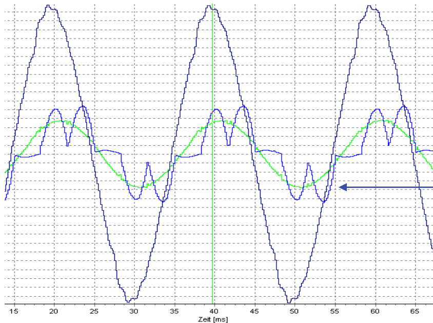
Netzspannung
